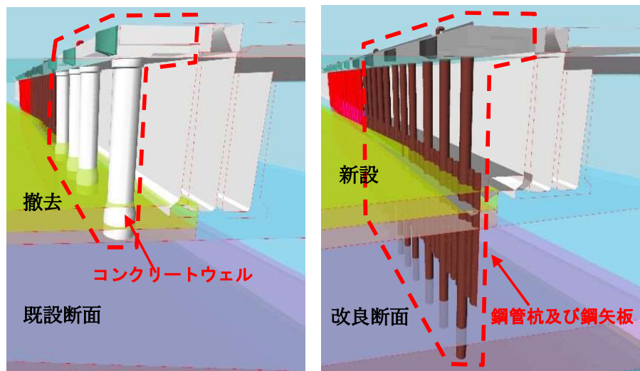
工事概要図
