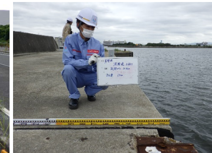
被災状況調査 (岸壁の変位等計測)
